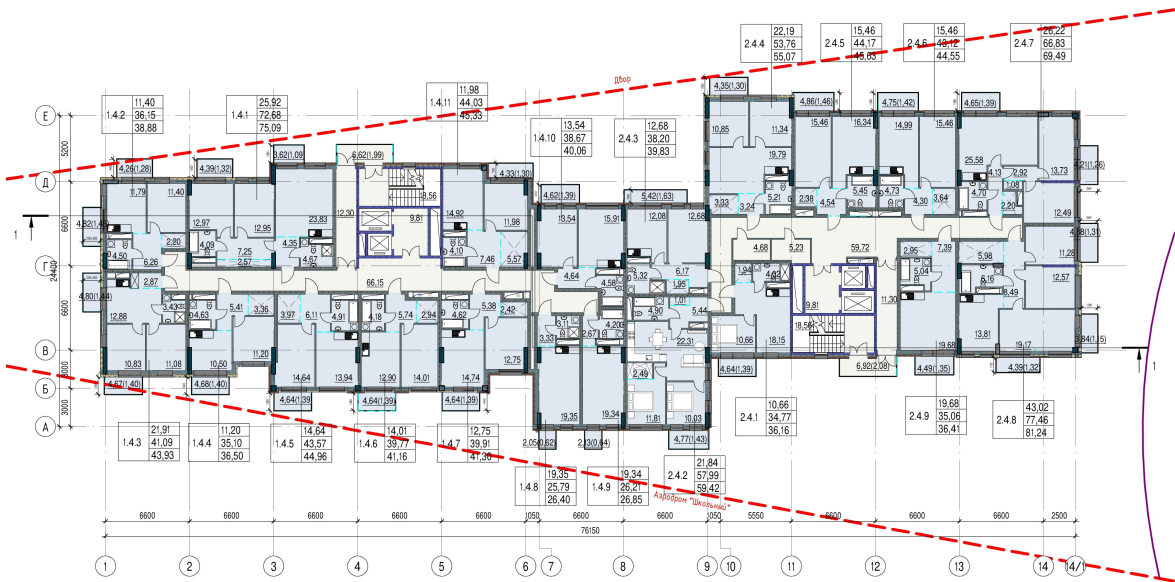
План 4-го поверху на відм. +10,650 (Черга І) М 1:200
